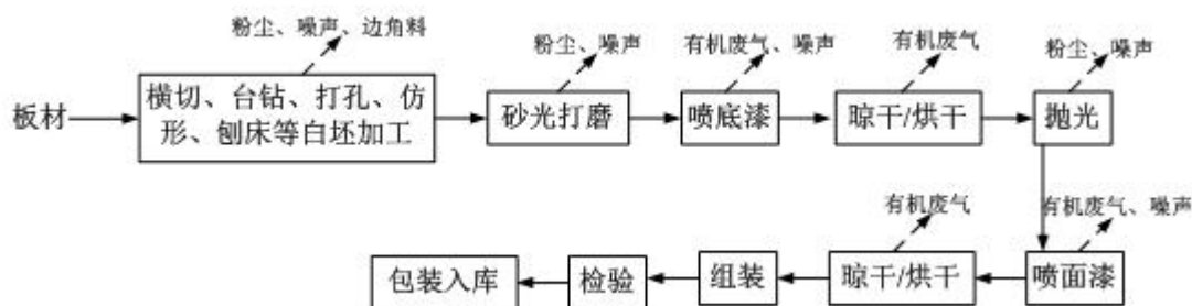
图 3-3 项目生产流程图
